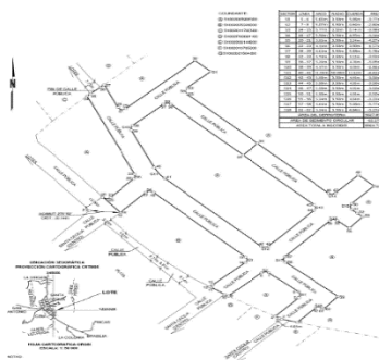
Figura N° 5. Plano de terrenos donado a la Municipalidad de La Cruz para la implementación de calles públicas en el distrito de Santa Cecilia
