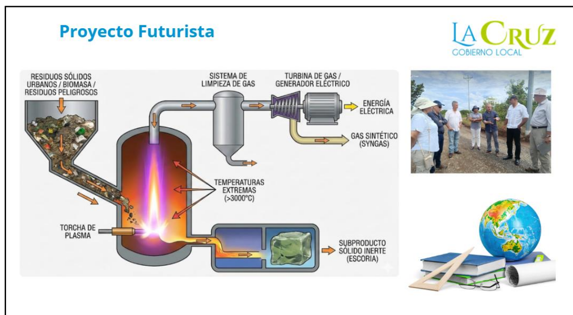
Figura N° 81. Esquema Técnico del Proceso de Gasificación por Plasma y Generación de Energía a partir de Residuos
